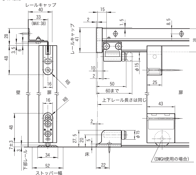
寸法図
